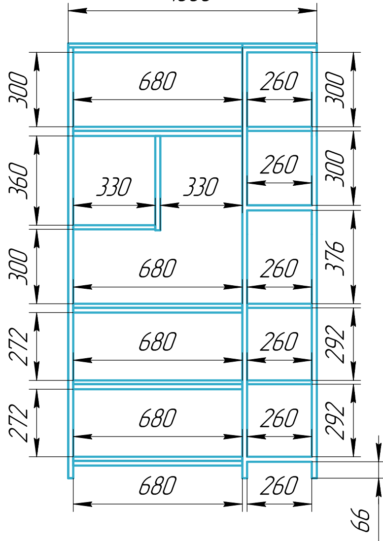
Вид Б 1000
