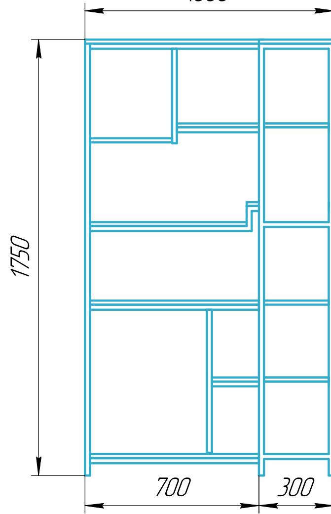
Вид Г 1000
