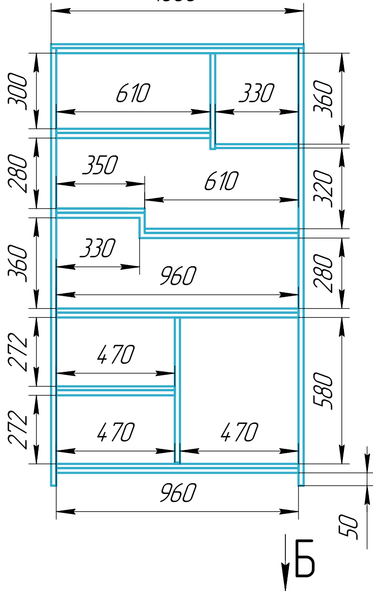
Вид А 1000
