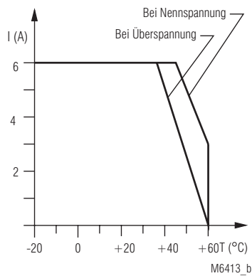
Dauerstromgrenzkurve
