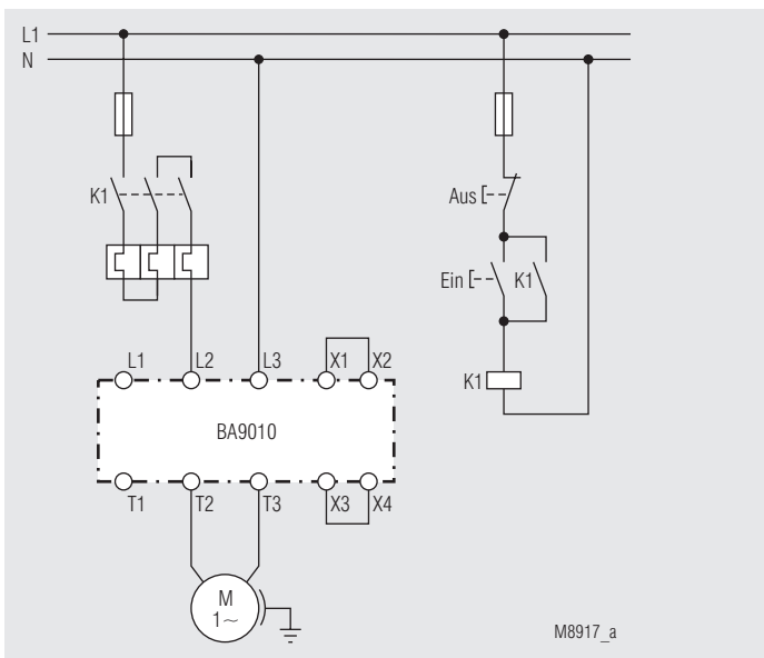
Sanftanlauf eines 1-Phasen-Motors an 230 V Wechselfspannung
